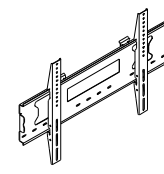
Bildschirmhalter 37 bis 70 Zoll VESA-Norm 200-600 max. Tragkraft 50 kg
